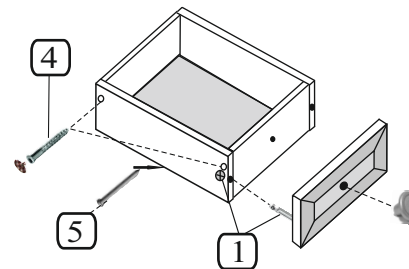
Схема сборки ящика
