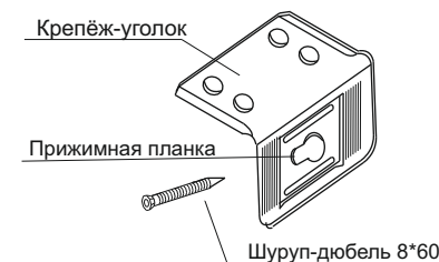
Крепление к стене
