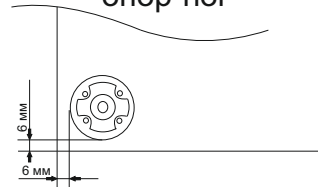
Схема присадки опор-ног
