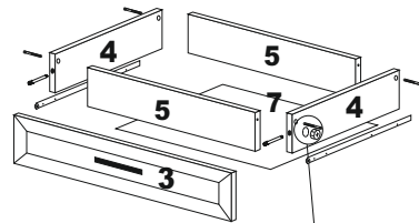
установка эксцентриковых стяжек
