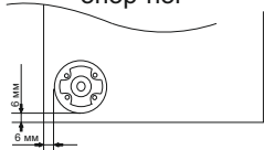
Схема присадки опор-ног
