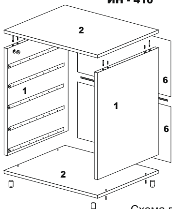
Схема присадки опор-ног
