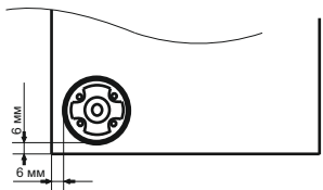
Схема присадки опор-ног
