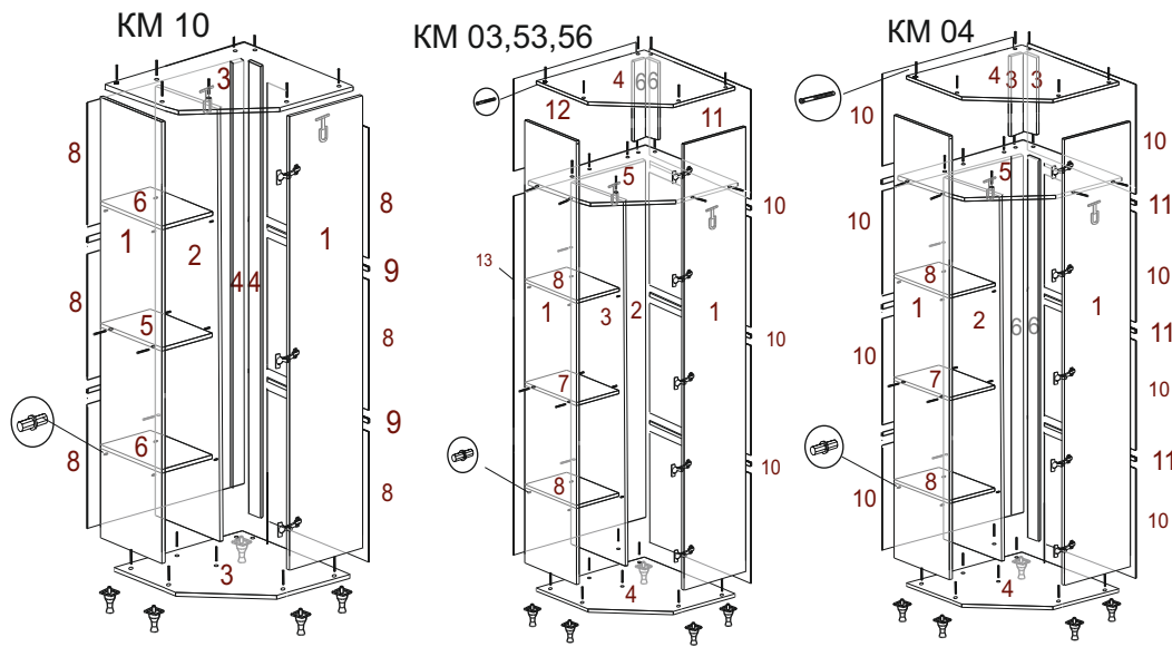
Схема присадки опор-ног
