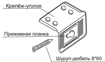
Крепление к стене
