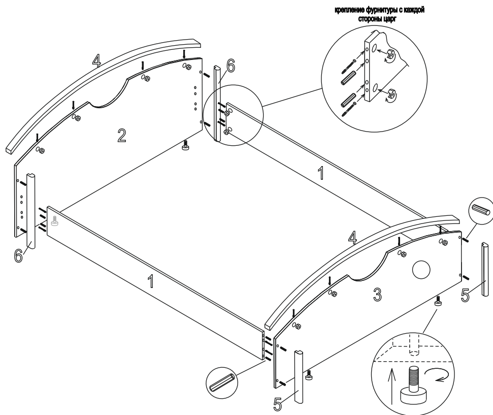
Комплекующие детали кровати под матрац 2000*1600
