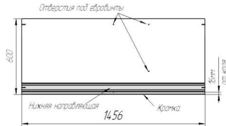
Рис.3 Схема установки нижней направляющей
