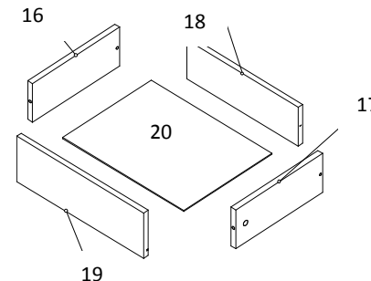
Рис.4 Схема сборки
