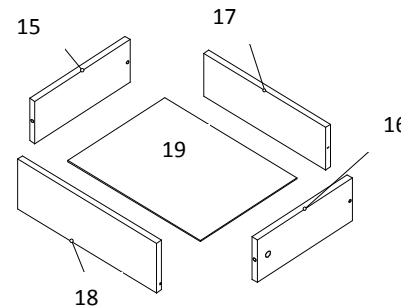
Рис.4 Схема сборки
